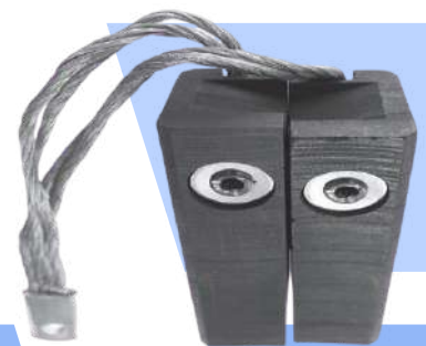
Escobilla NCR-012 Medidas 2.500 x 1.000 x 1.250 in EG
